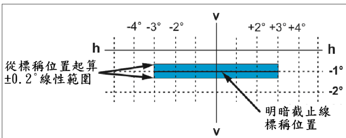
圖三：明暗截止線形狀和位置
