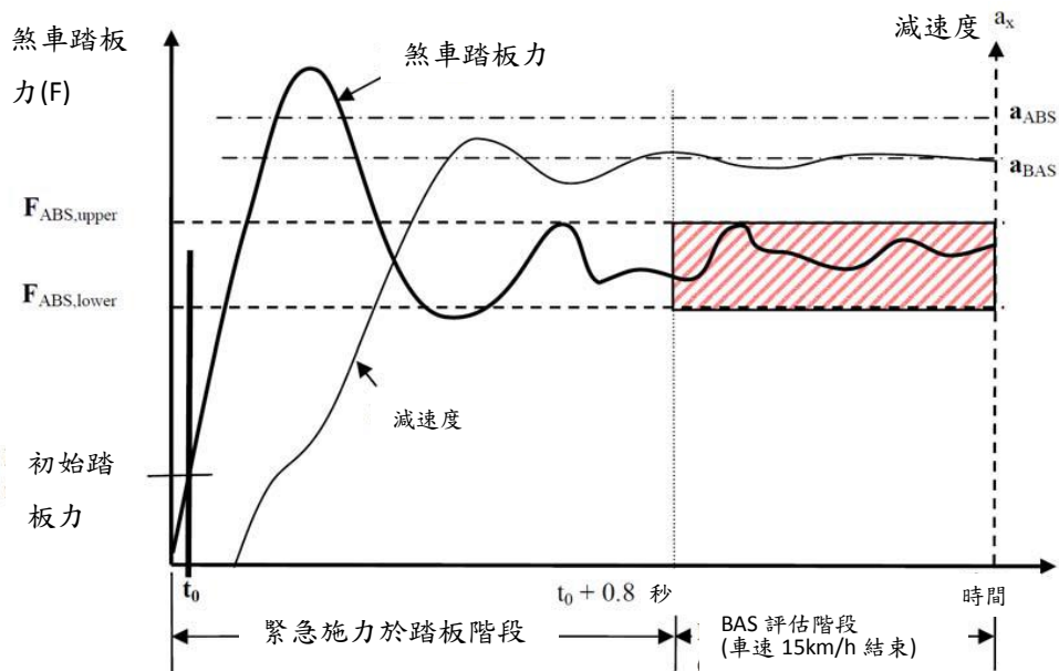
圖九、B類BAS系統之試驗二圖例
