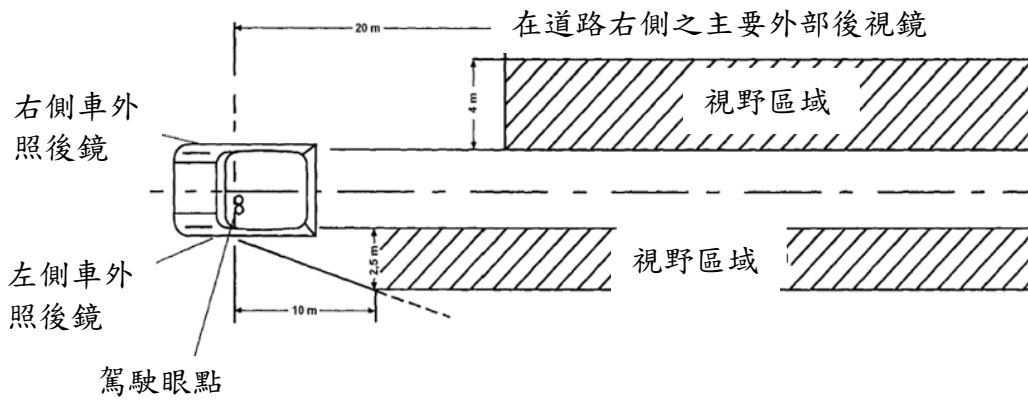
圖八：VII類主要後方視鏡之地面視野區域
