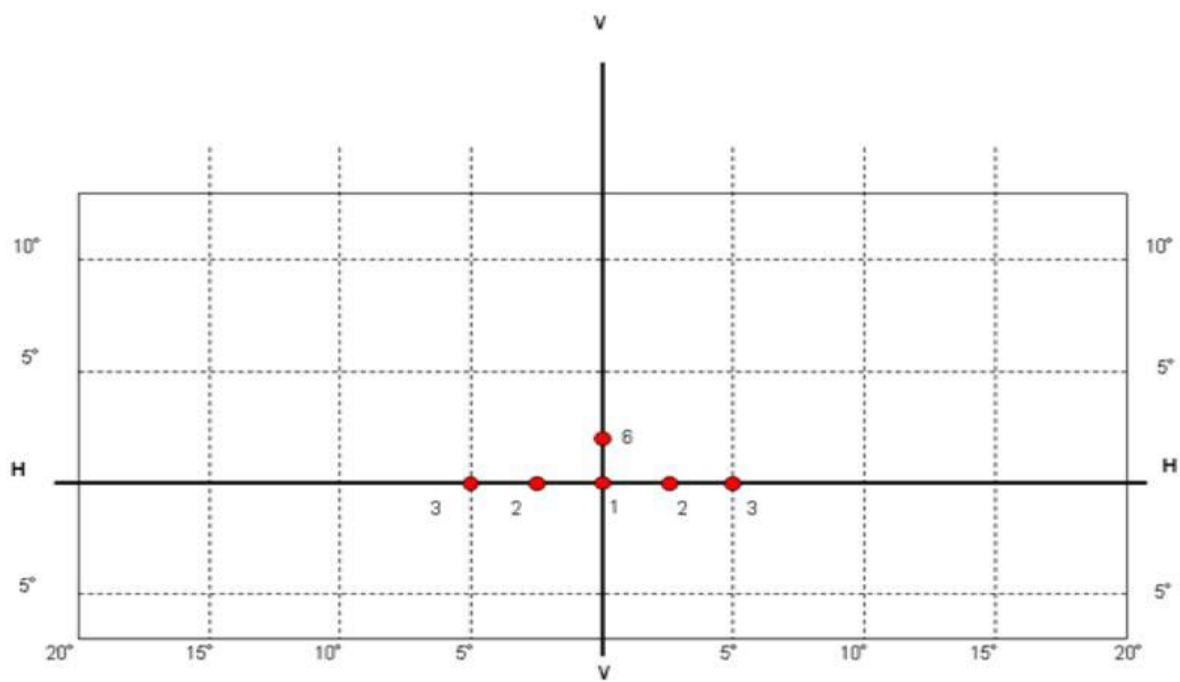
圖一一：類型 E 對稱光型次要遠光光束之測試點位置
