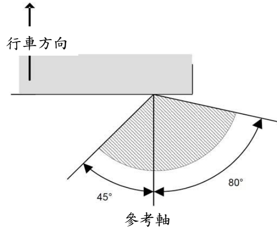
圖二：尾燈(適用 4.6.1 之 M/N/O/L 類車輛及 4.6.2.2 之 L 類車輛)
