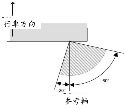
圖二之一：安裝後車輛尾燈之 H 平面距地高不超過七五〇公釐者角度(適用 4.6.1 之 M/N/O/L 類車輛)
