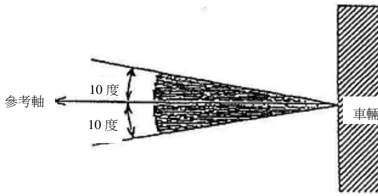
圖二 SM2 光度分佈
