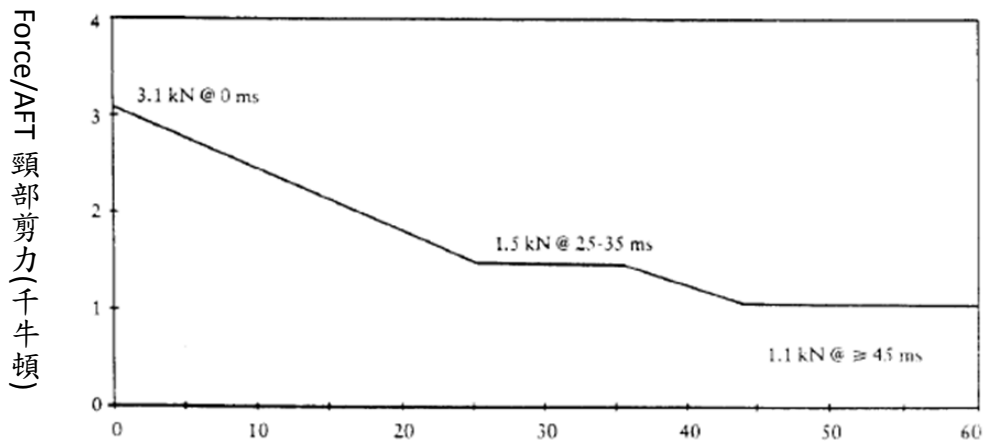
圖二：頸部剪力標準
