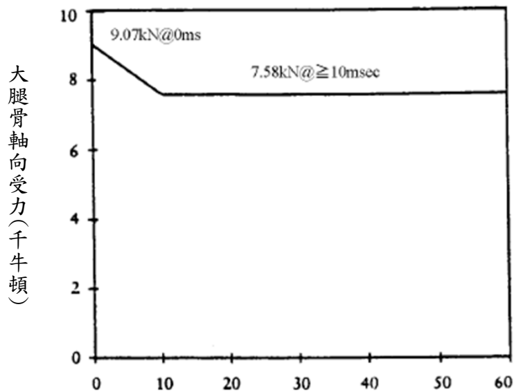
圖三：大腿骨受力標準
