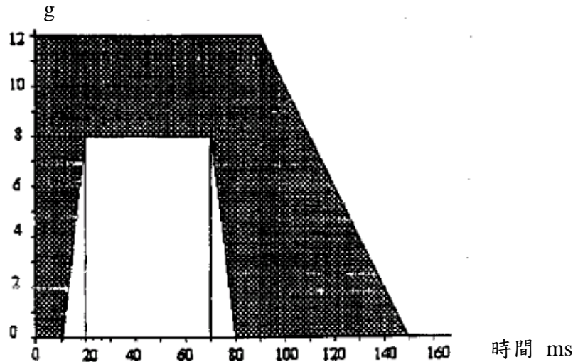
圖五：台車衝擊時之減速度或加速度
