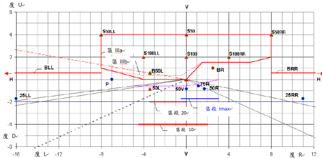
圖一：近光光束光度量測點
