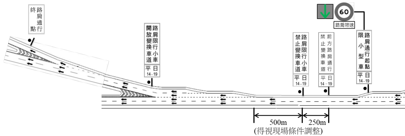
附圖 1：開放路肩終點銜接出口減速車道或出口匝道示意圖
