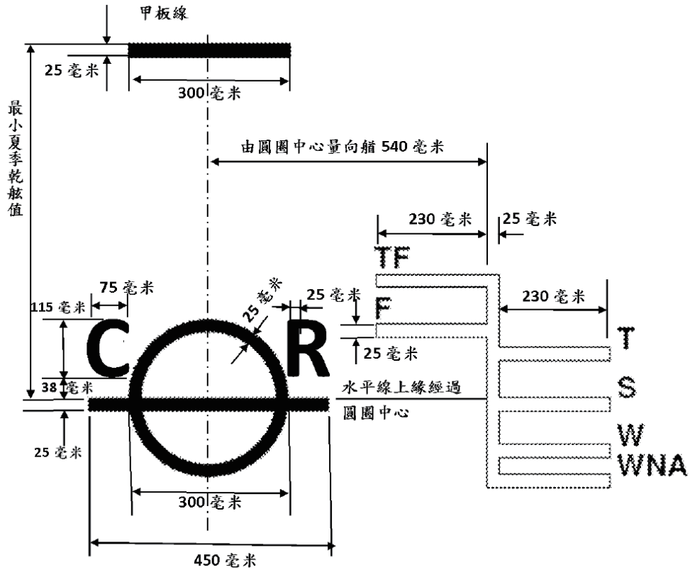
附圖二 國際航線船舶載重線所使用之各線標
