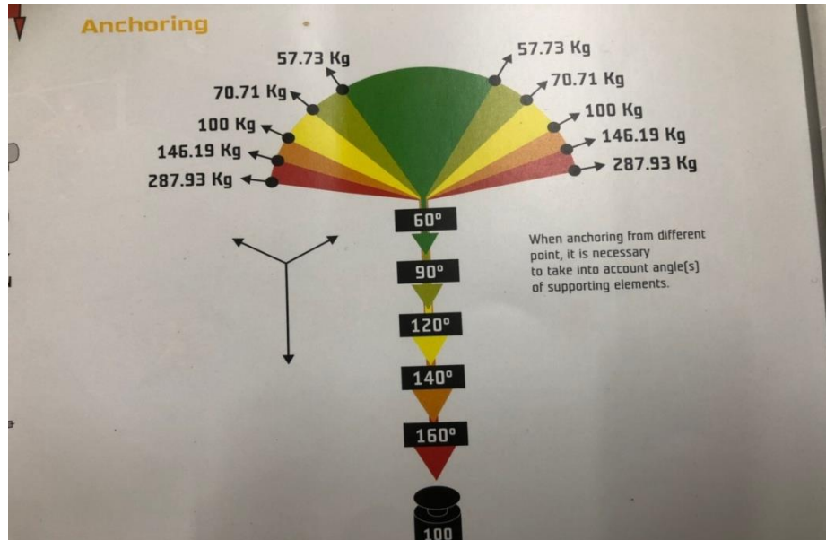
圖 3：Y 型架設各內角角度造成之繩張力。
