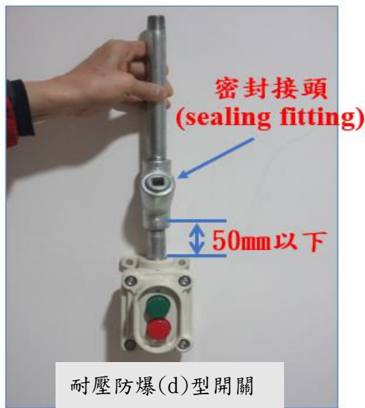
圖 5 耐壓防爆電氣設備應在距離接口處 50mm 範圍內裝設密封接頭例
