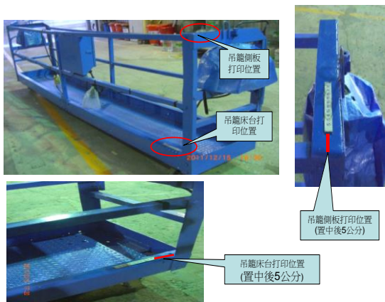
附圖 2-1：吊籠工作床台打印位置
