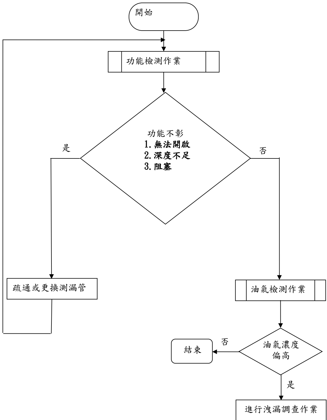
圖1 土壤氣體監測作業整體流程圖
