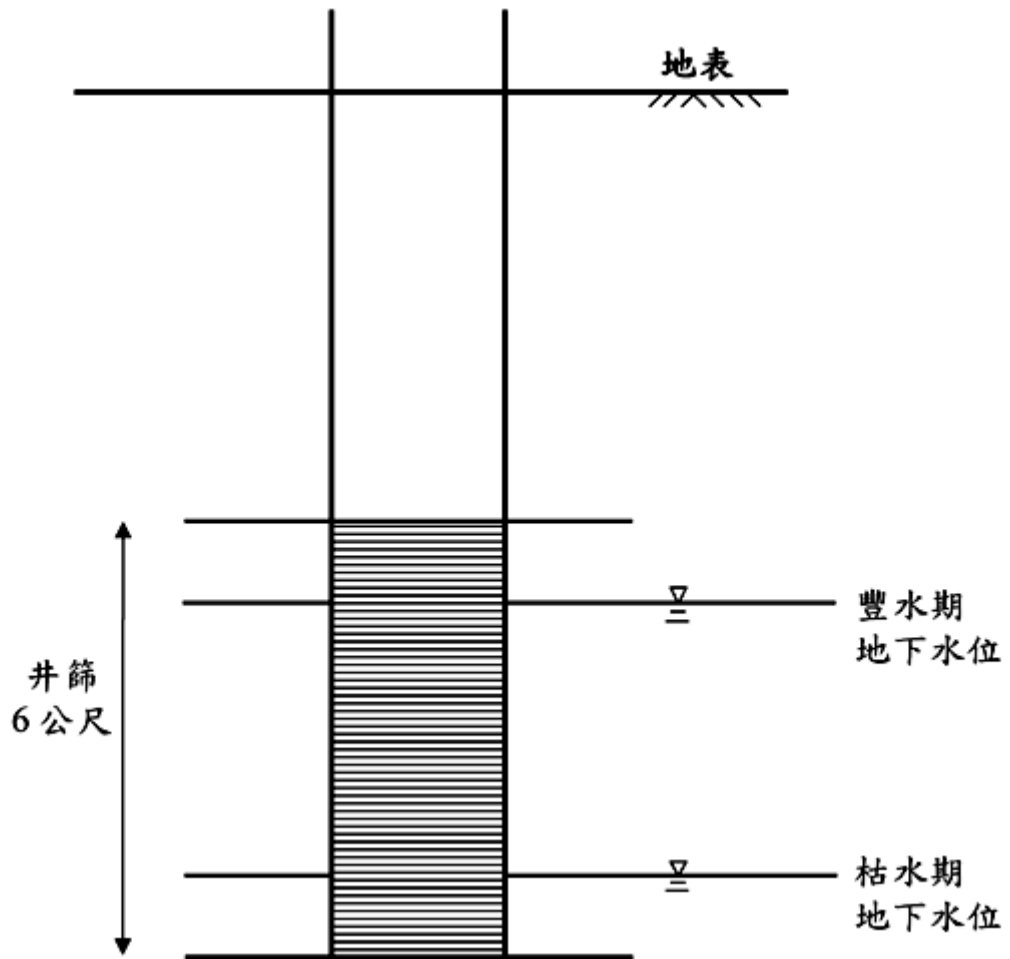
圖2-3 非受壓含水層在豐水期和枯水期鑽孔深度及井篩位置示意圖（未按比例）
