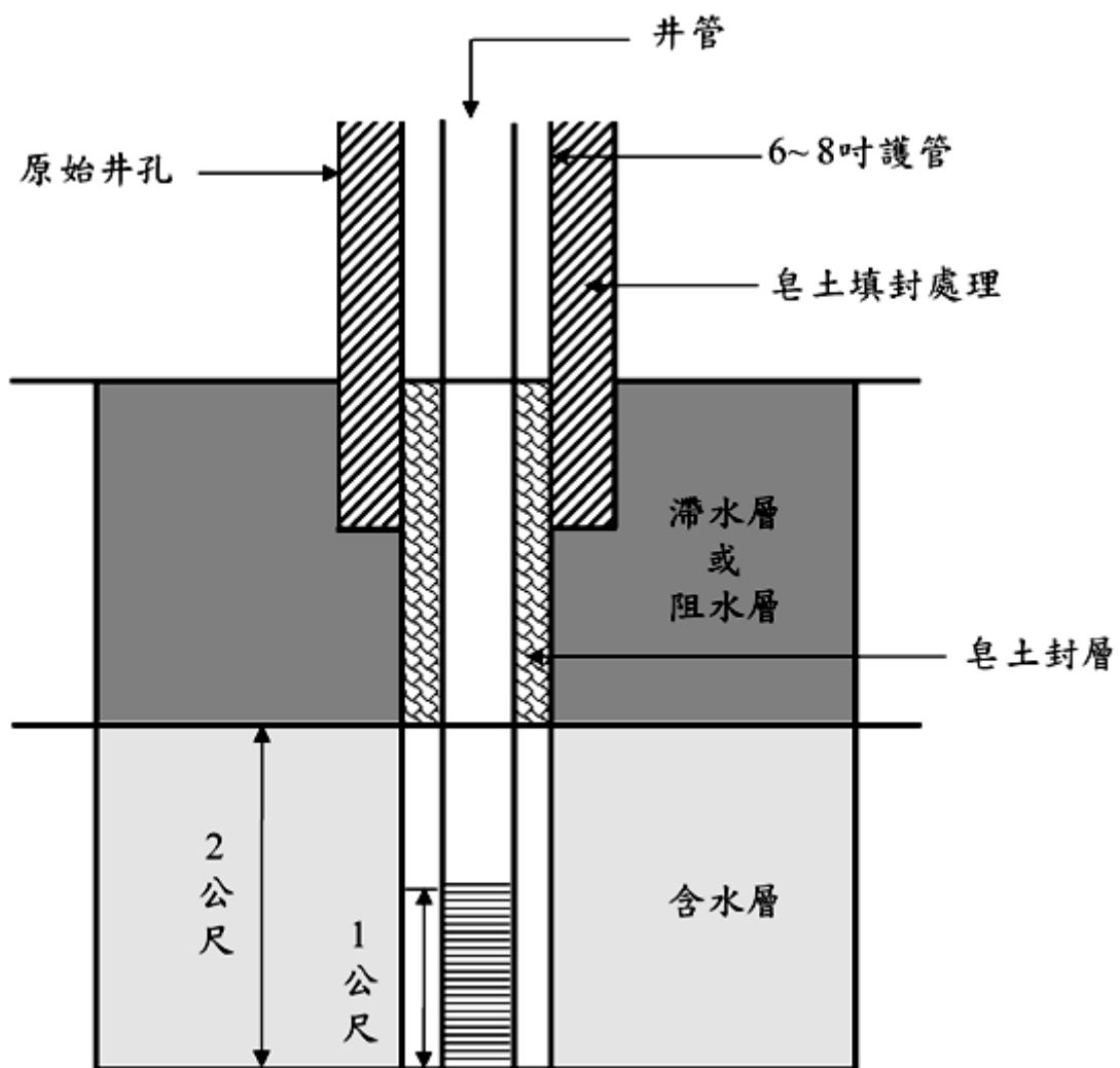
圖2-4 貫穿受壓含水層覆蓋時防止錯接污染措施示意圖（未按比例）
