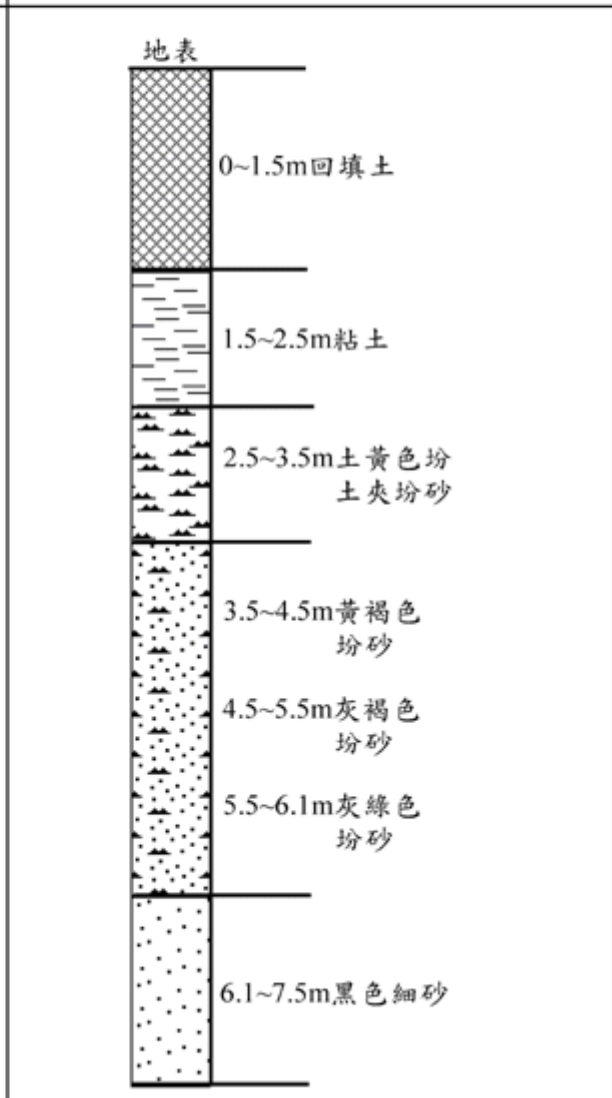
地質剖面圖
