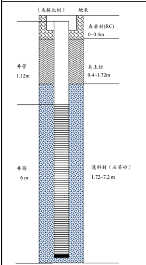
監測井構造圖
