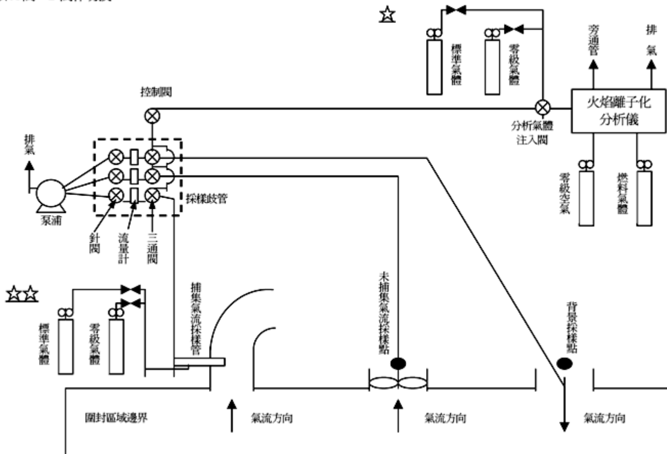
圖1 TVOC濃度量測系統配置示意圖
