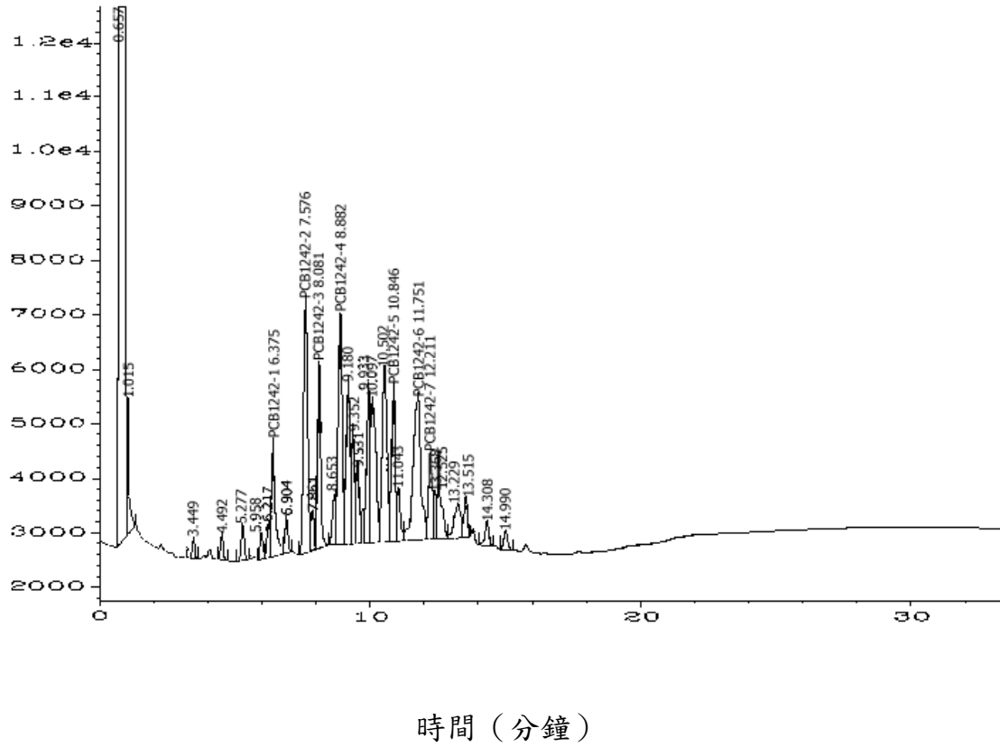
圖一 多氯聯苯標準品 (Aroclor-1242) 氣相層析圖譜 (DB-1管柱)
