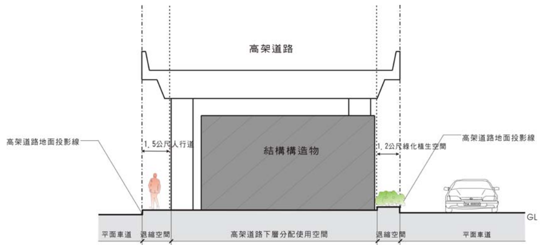
附圖四:高架道路下層構造物退縮1.5公尺人行道 或1.2公尺綠化植生空間剖面示意圖
